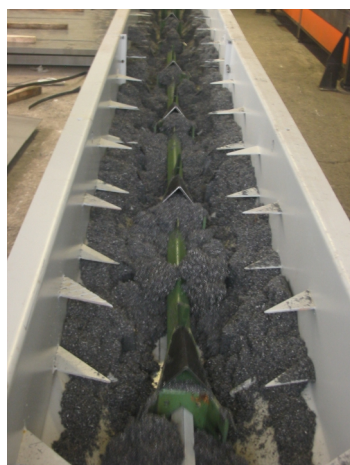
Linea ad arpioni trasporto trucioli corti
