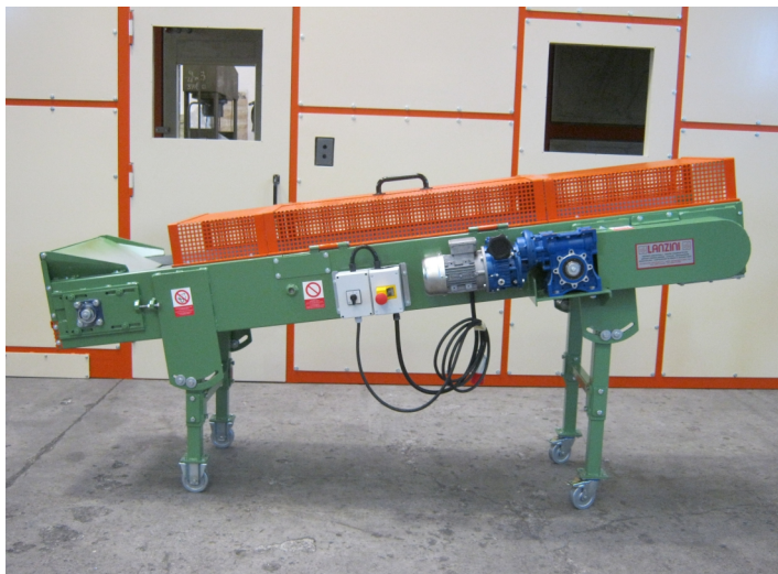
Trasportatore a tapparelle per pezzi stampati caldi
