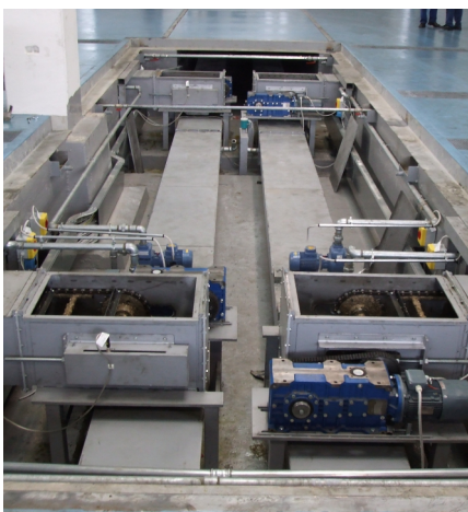
Linea centralizzata a pale draganti
